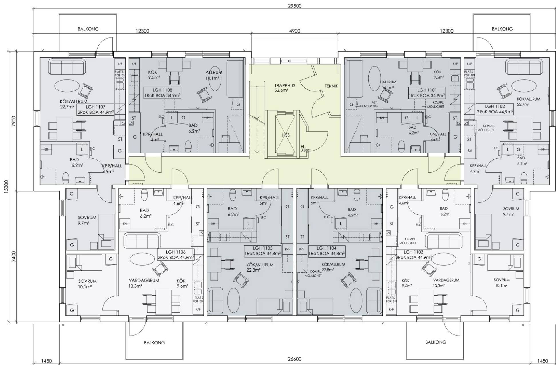
NORMALPLAN Våning 1-5 SKALA 1:100
