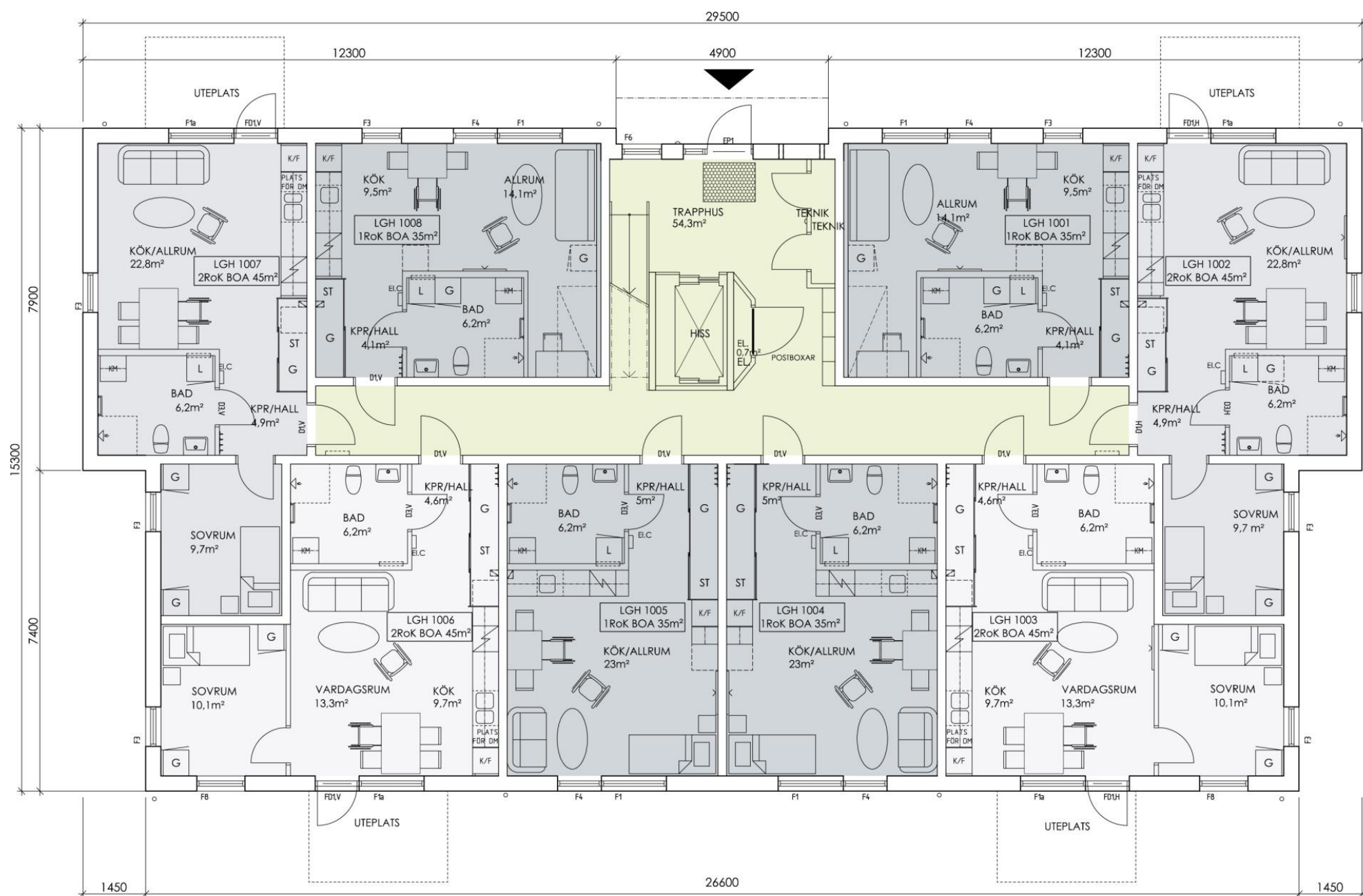
ENTRÉPLAN SKALA 1:100
